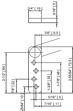
Jamb Bracket
